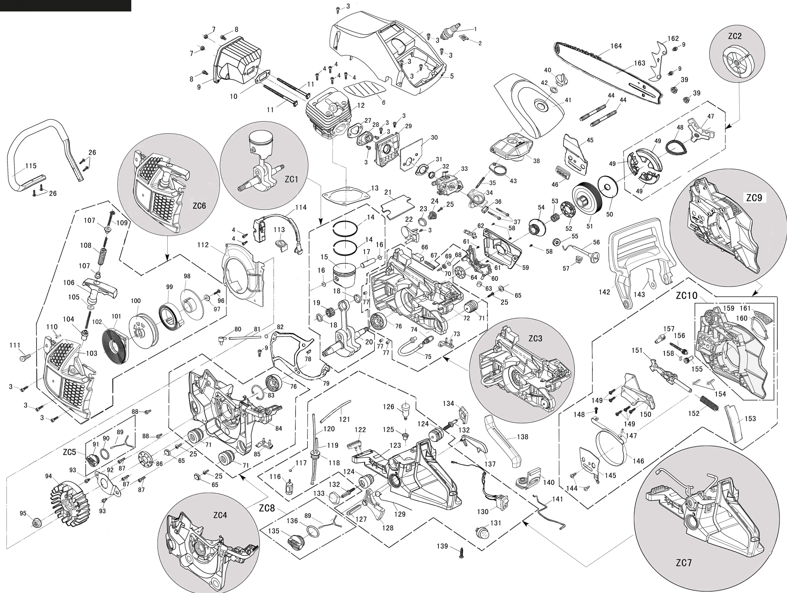
51.06-PRB-45-51 PILA ŘETĚZOVÁ BENZINOVÁ 50.8CCM, LIŠTA 45CM
